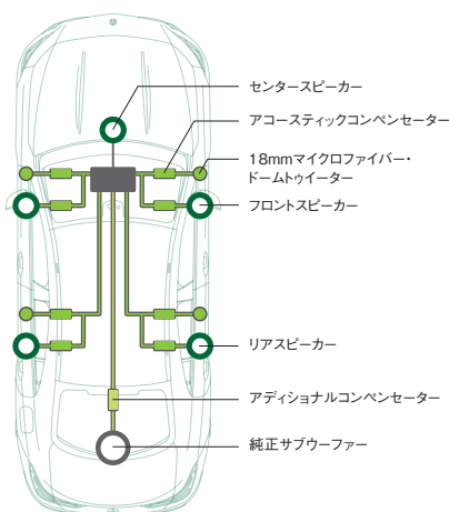
システム構成図 ※イラストはCLAクーペ
